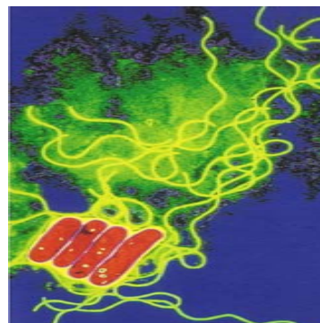
Legionella Bacteria
